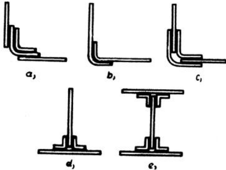
Sarokkötések
