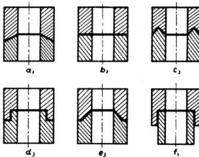
Ragasztott csőkötések
