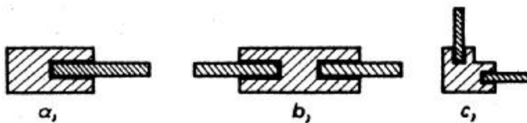
Hornyolt kötések
