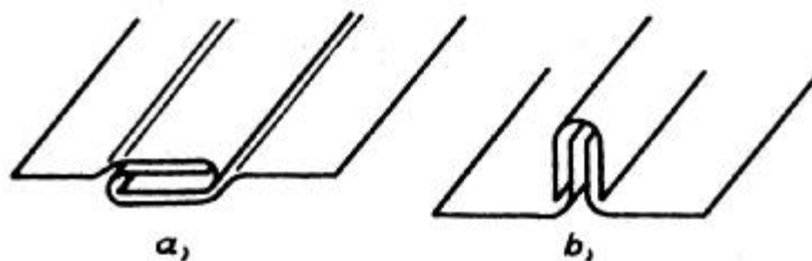
Hajtogatott kötések
