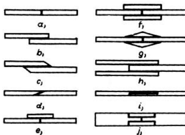
Ragasztott lemezkötések
