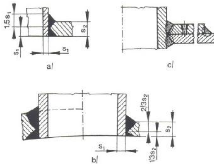
Csőcsatlakozások
