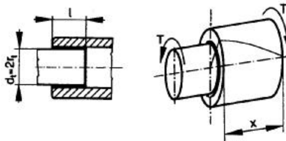
Nyomatékkal terhelt ragasztott kötés
