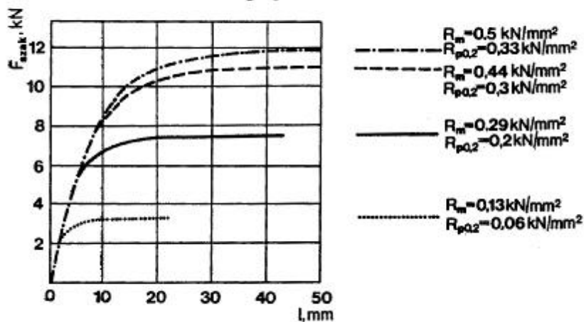
A terhelhetőség és az átlapolási hossz kapcsolata
