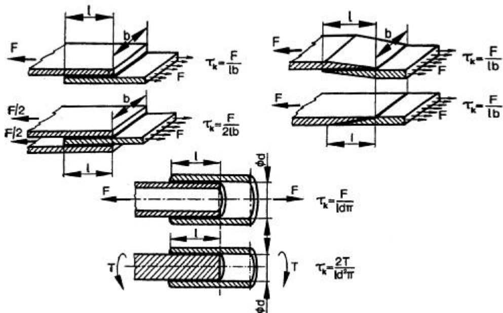
Az átlagos nyírófeszültségek
